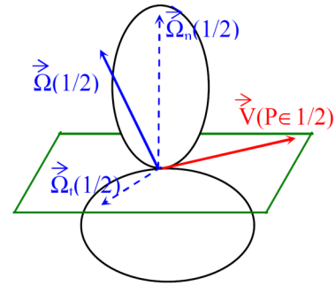
Contact ponctuel entre les solides 1 et 2
